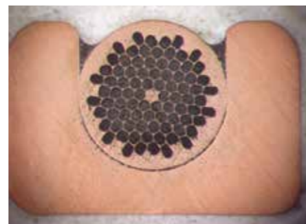
MRI 槽芯线 (WIC) 84芯超级超导导线
